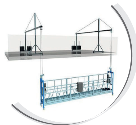
Plates-formes suspendus motorisées ou échafaudages volants
